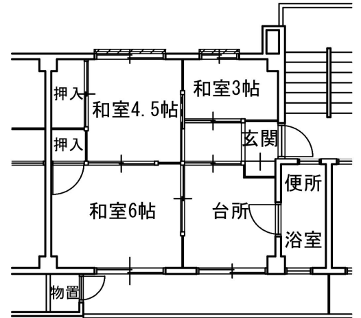
代表間取図（左右反転タイプあり）
